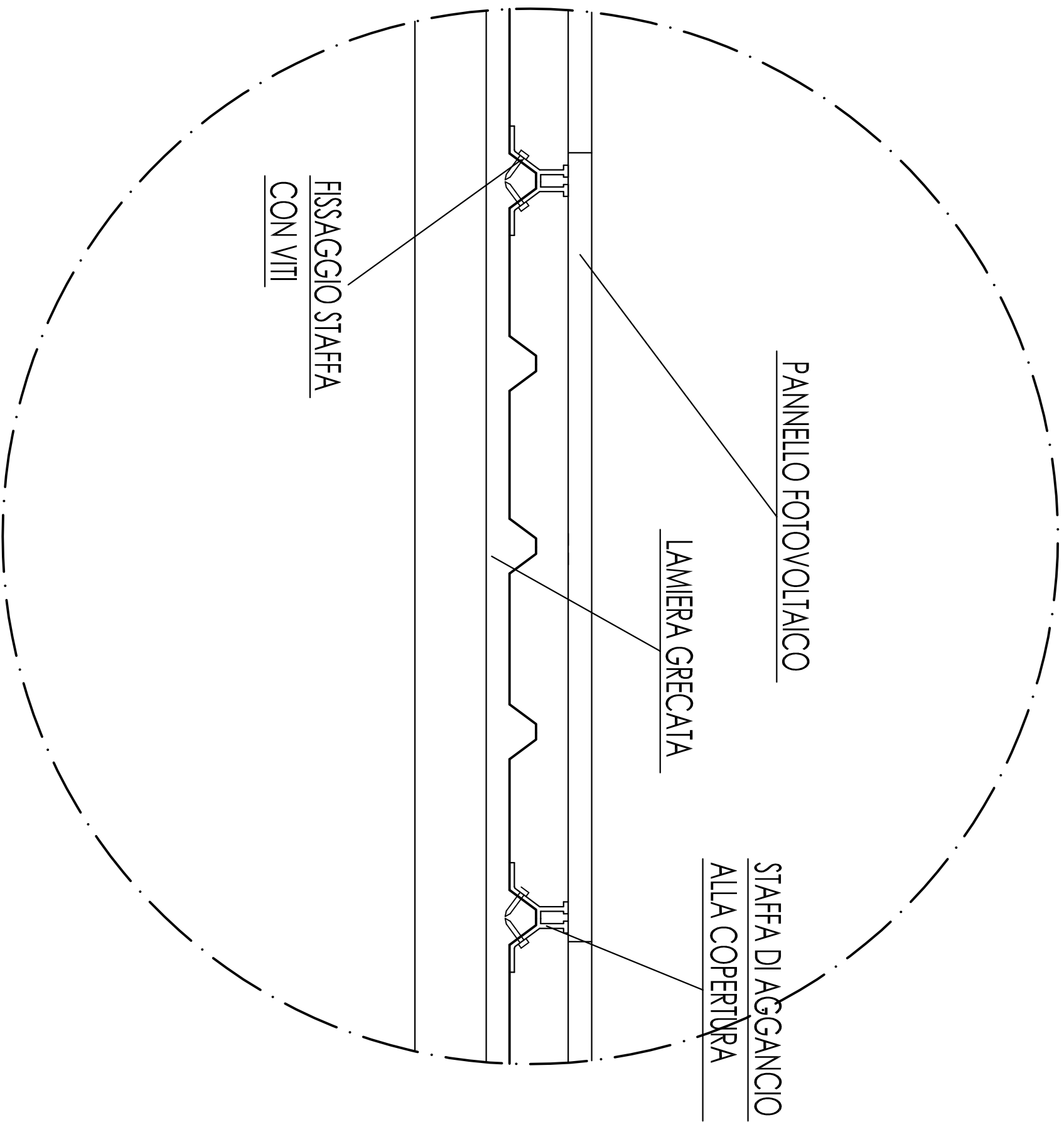
PARTICOLARE AGGANCIO DEL PANNELLO FOTOVOLTAICO ALLA COPERTURA scala 1:10
